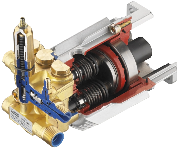
Taumelplattenpumpe
