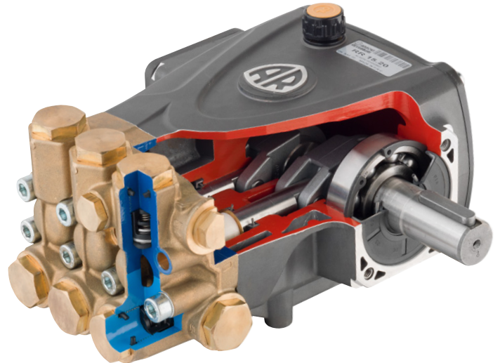
Kurbelpumpe
