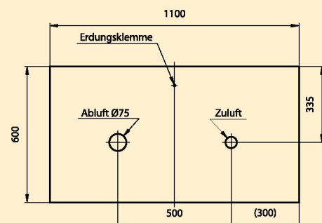
Rückansicht VBF.60.110-S und VBF.60.11.5-S VBF.60.110-2S und VBF.60.11.5-2S VBF.60.110-T und VBF.60.11.5-T VBF.60.110-A und VBF.60.11.5-A
