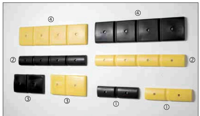
Hohe Eckschutzprofile (H 500 mm) in Kombination mit breiten Wandschutzprofilen (H 250 mm)
