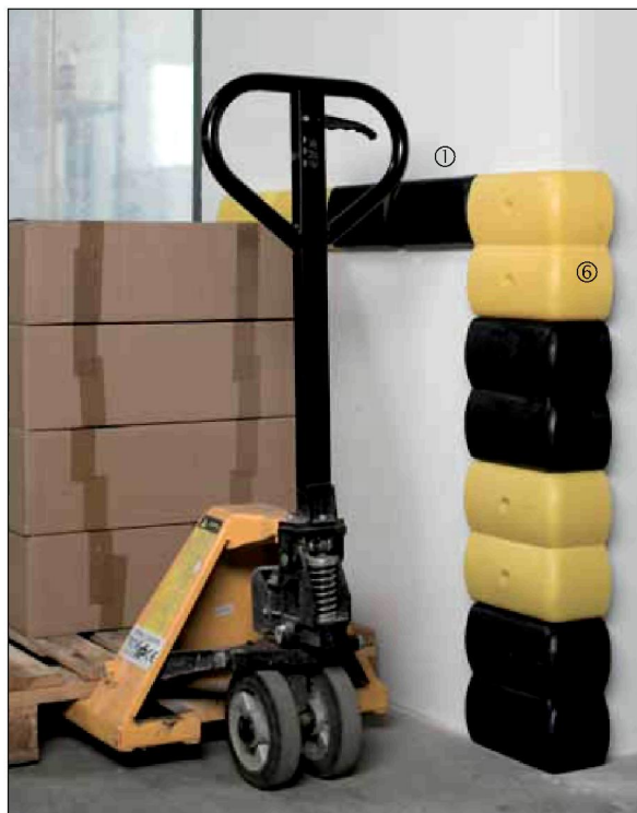
Eckschutzprofil (H 250 mm) in Kombination mit schmalen Wandschutzprofilen (H 125 mm)
